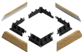
CHAPITEAU OU BASE DE COLONNE POUR COLONNES 7" ET 8"
